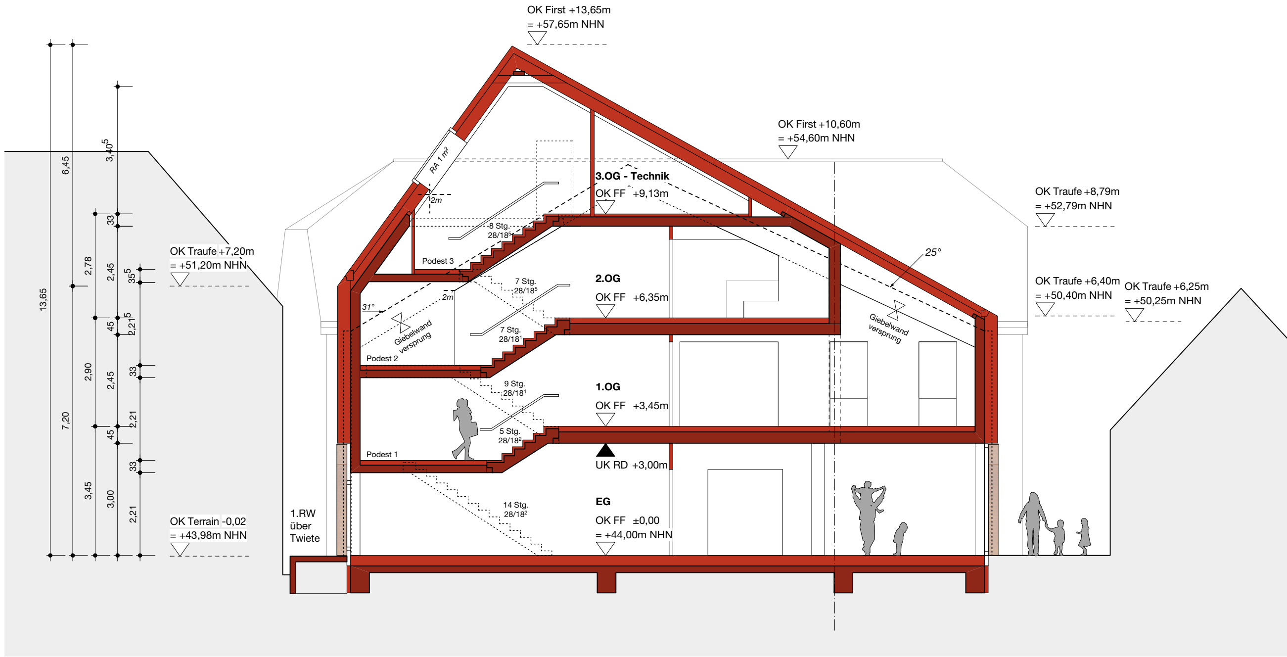
NEUBAU Schnitt E-E
