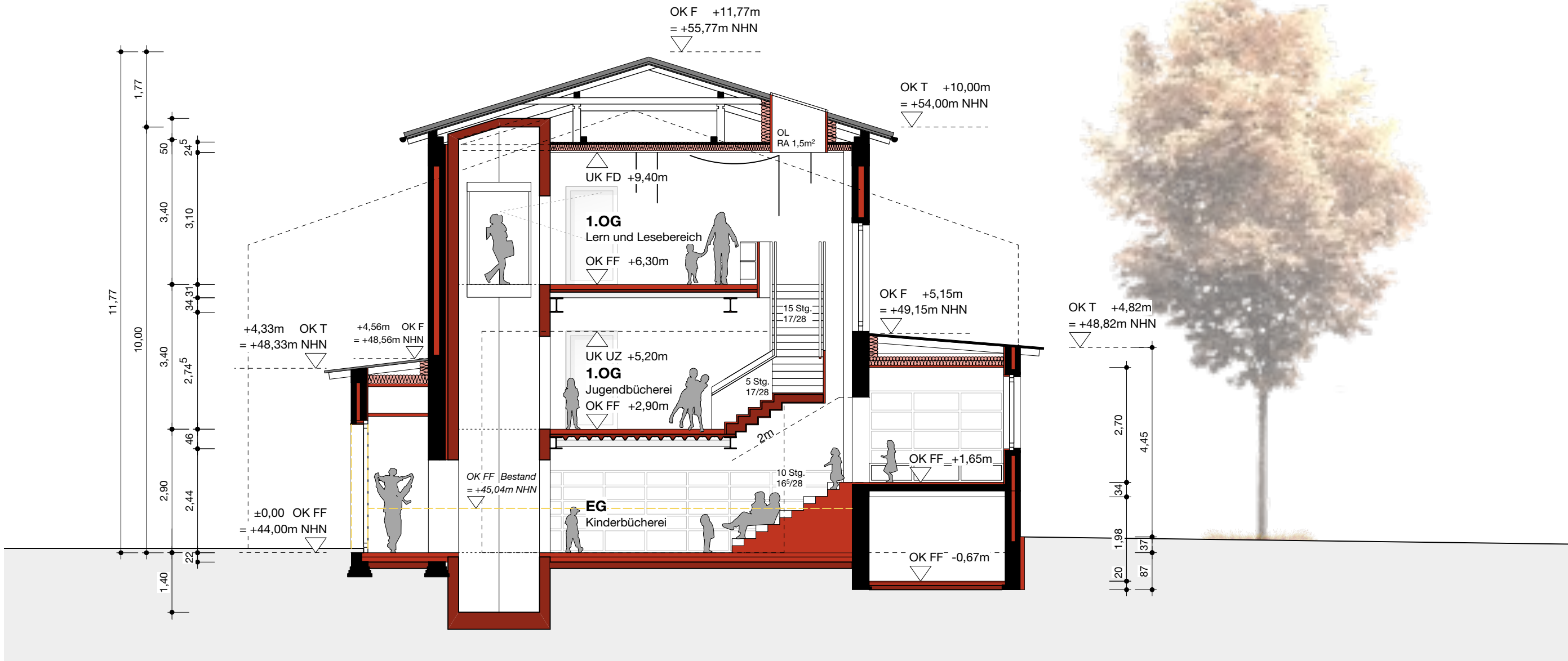
TURMGEBÄUDE Schnitt C-C
