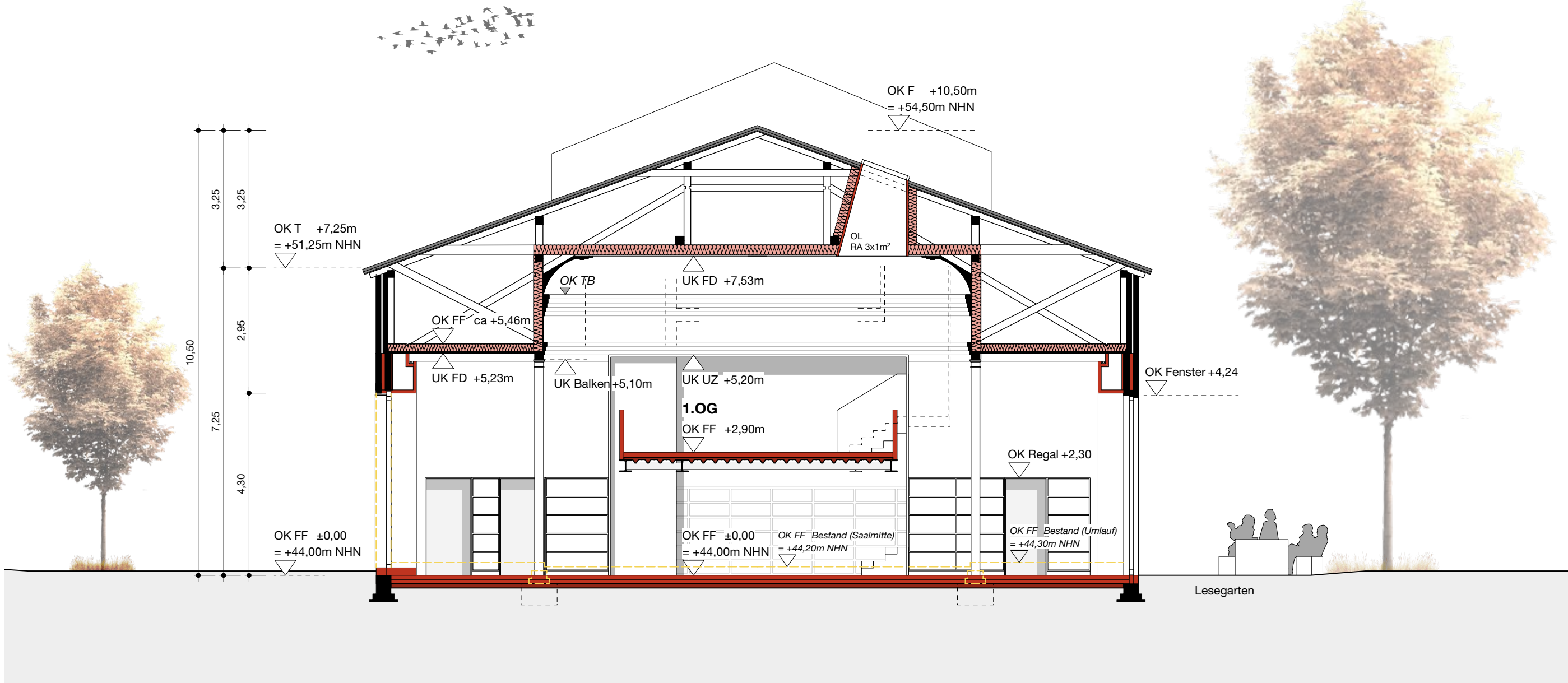
SAALGEBÄUDE Schnitt D-D
