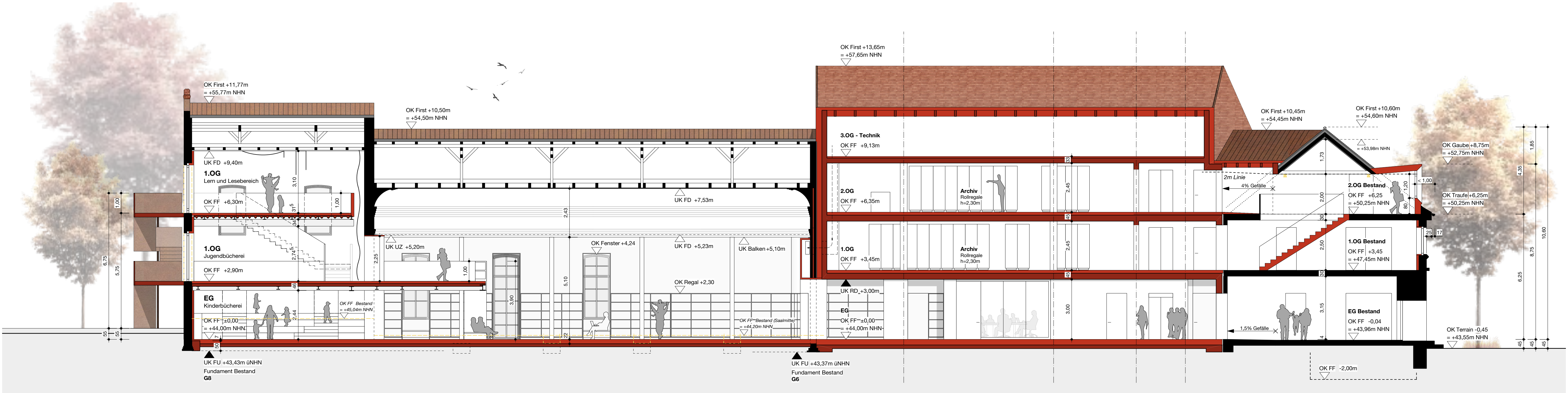
LÄNGSSCHNITT GESAMT Schnitt A-A
