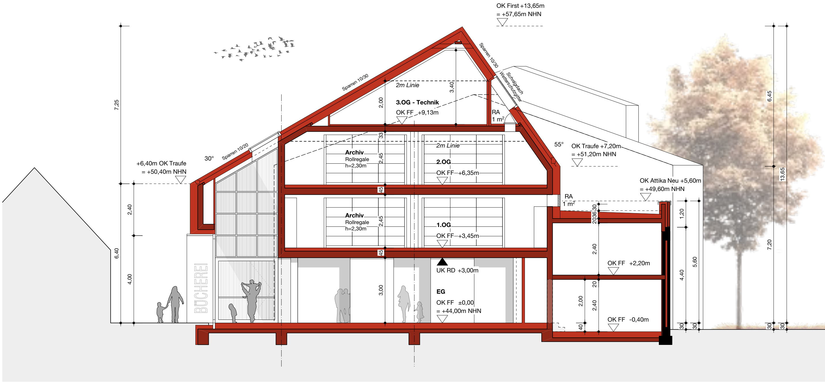
NEUBAU Schnitt B-B
