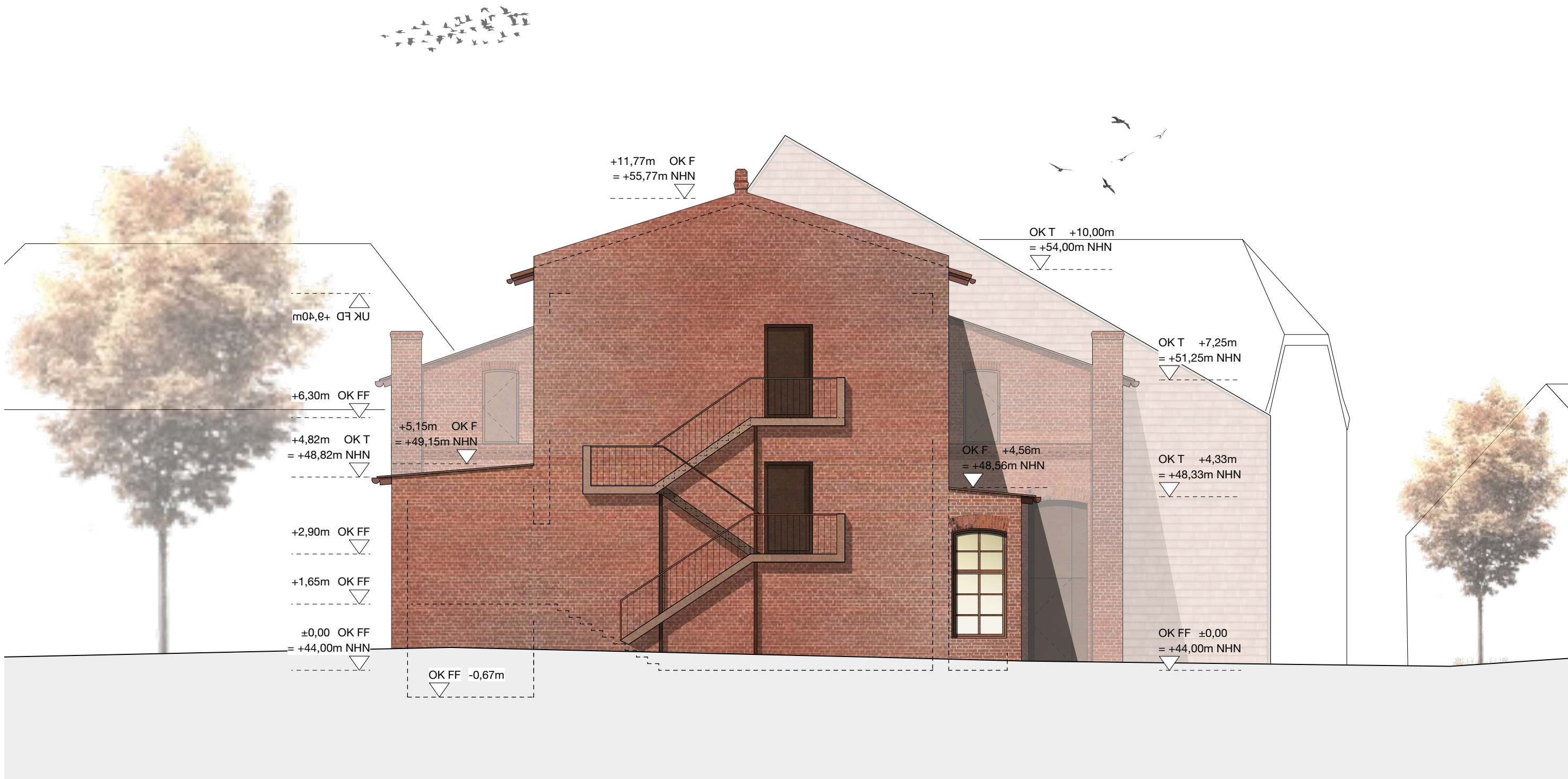
ANSICHT NORD
